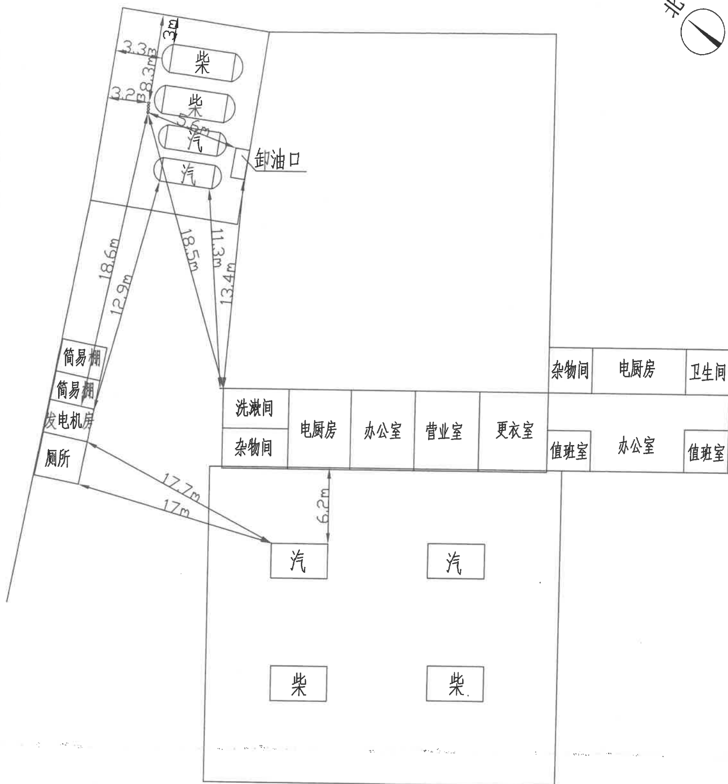
高阳县边渡口加油站（普通合伙）平面布置示意图
