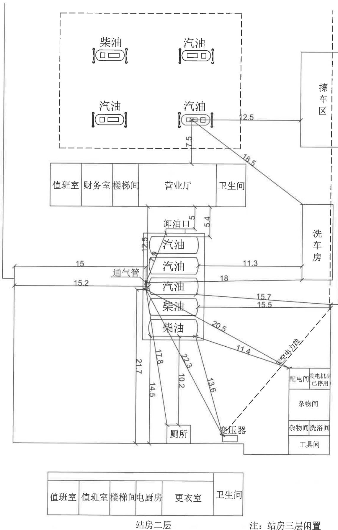
博野县博阳中博加油站平面布置示意图
