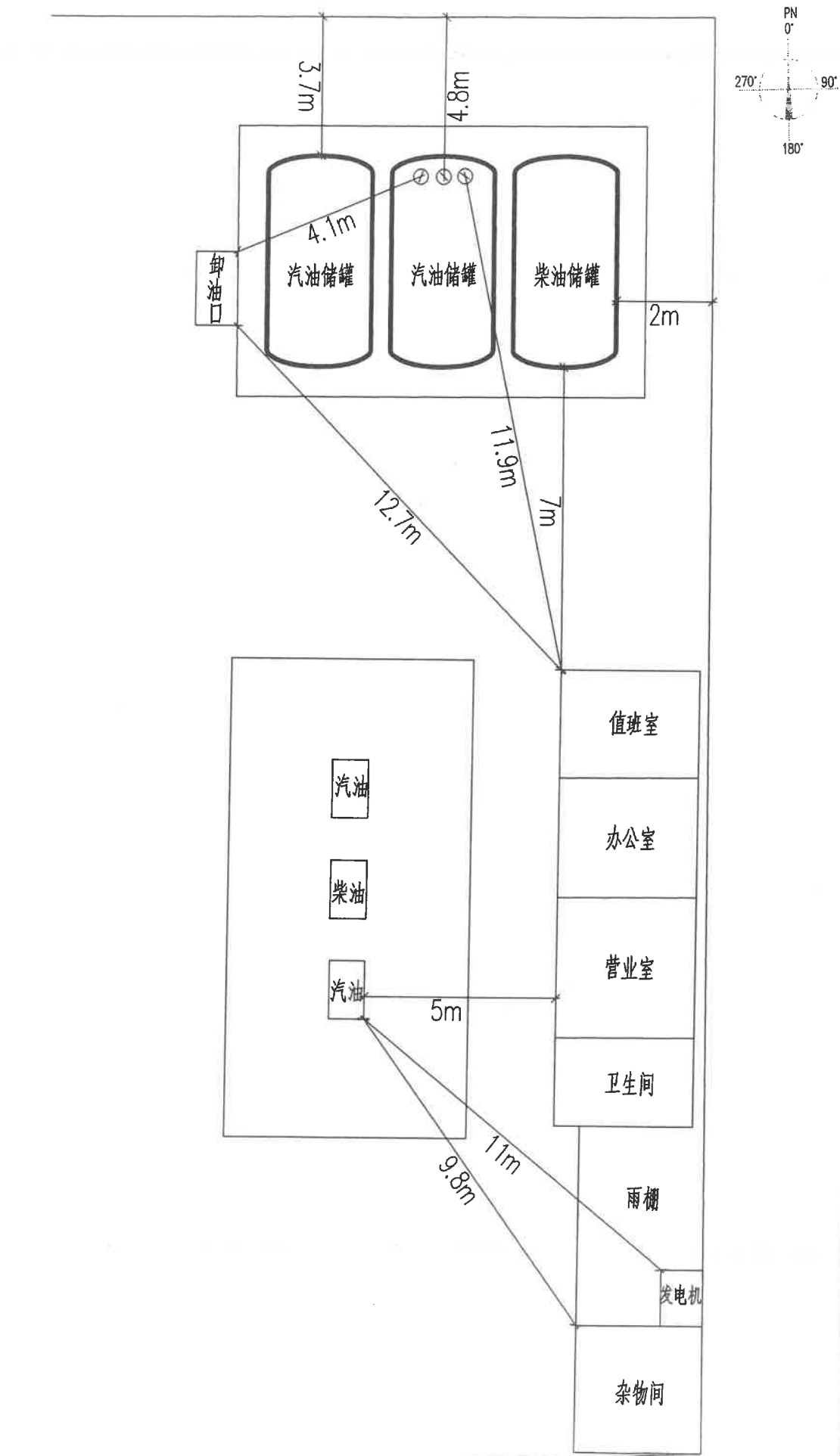
保定市博隆加油站(普通合伙)平面布置示意图
