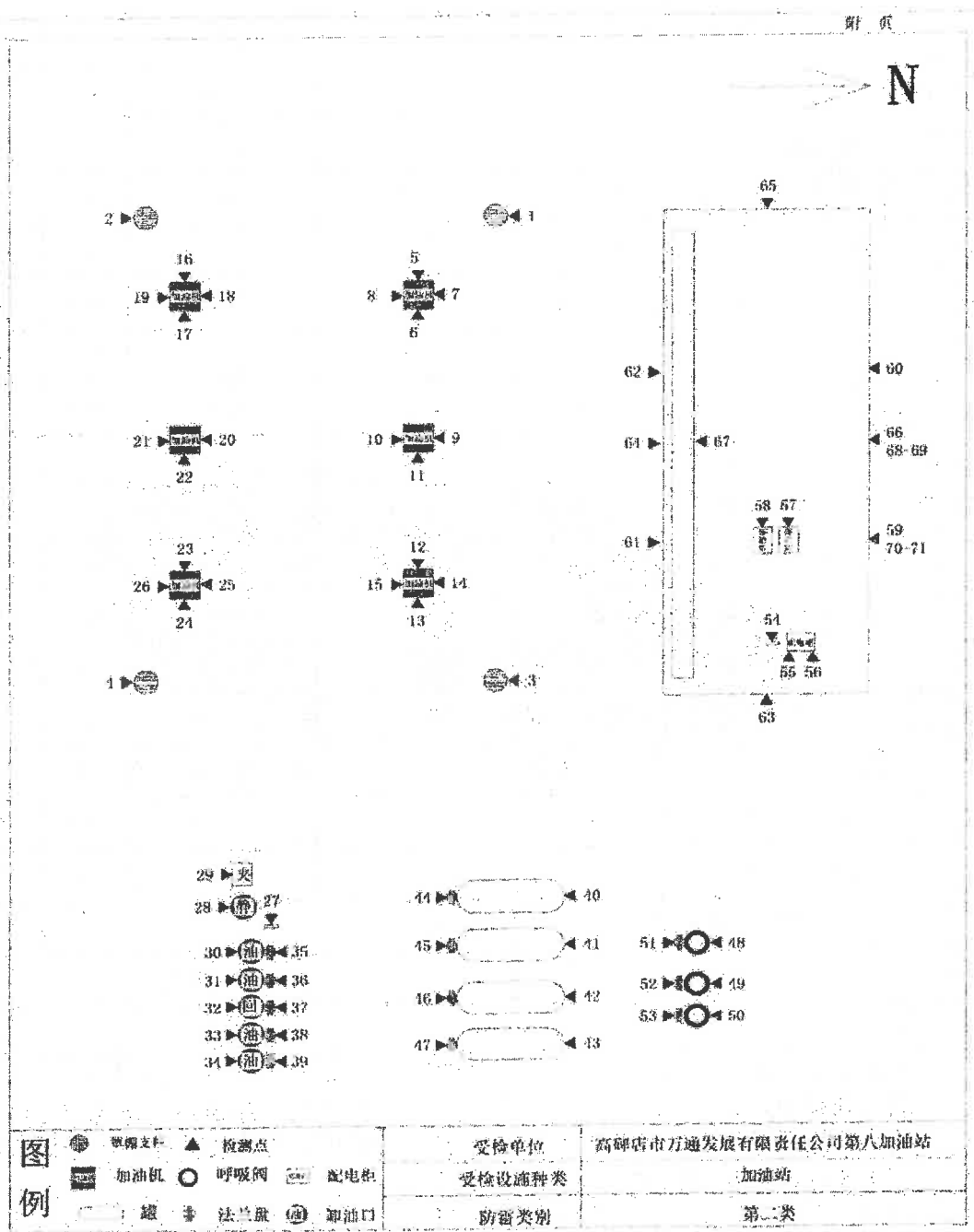
被保护物测点平面示意简图
