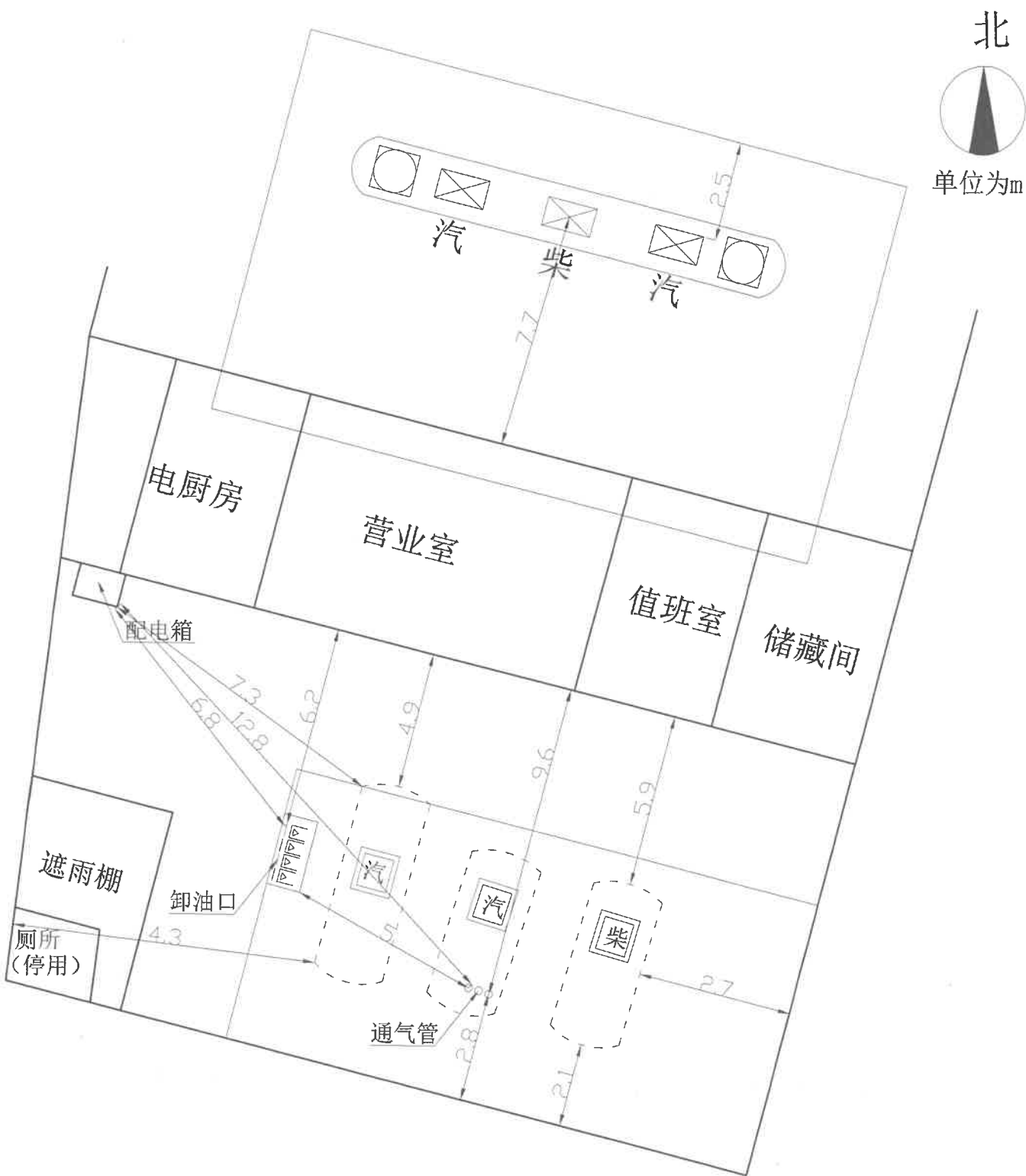
涿州市书恒加油站平面布置示意图
