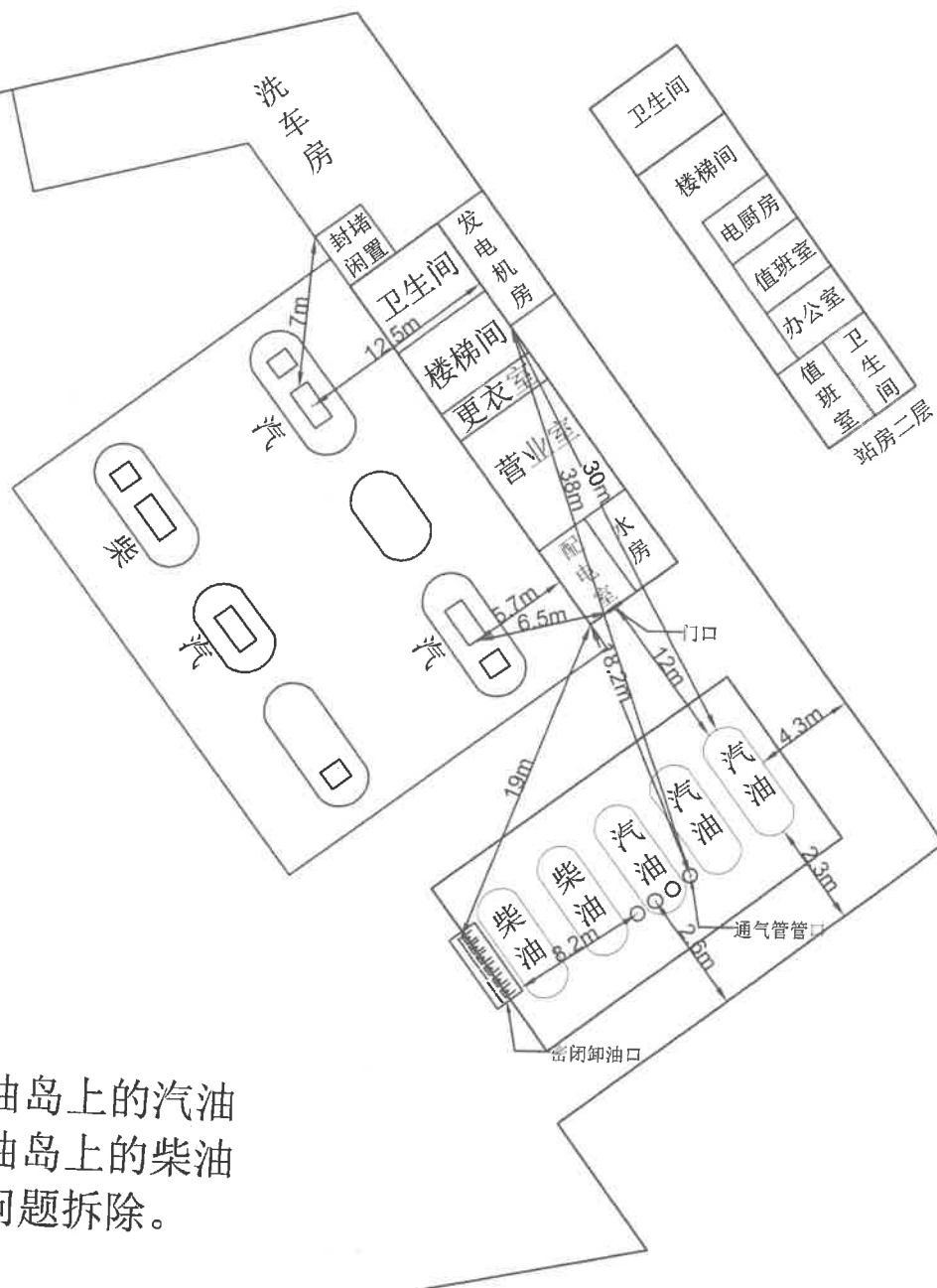
曲阳县京昆新能源科技有限公司 京昆加油站平面布置示意图
