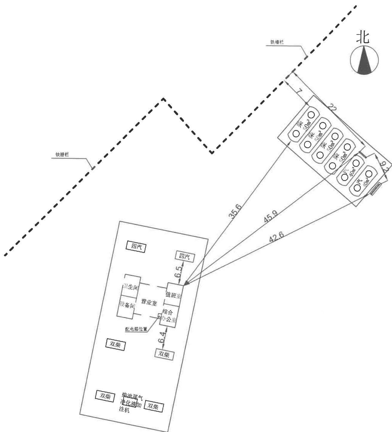
中国石油天然气股份有限公司河北保定销售分公司 第一百八十九东区加油站平面布置示意图
