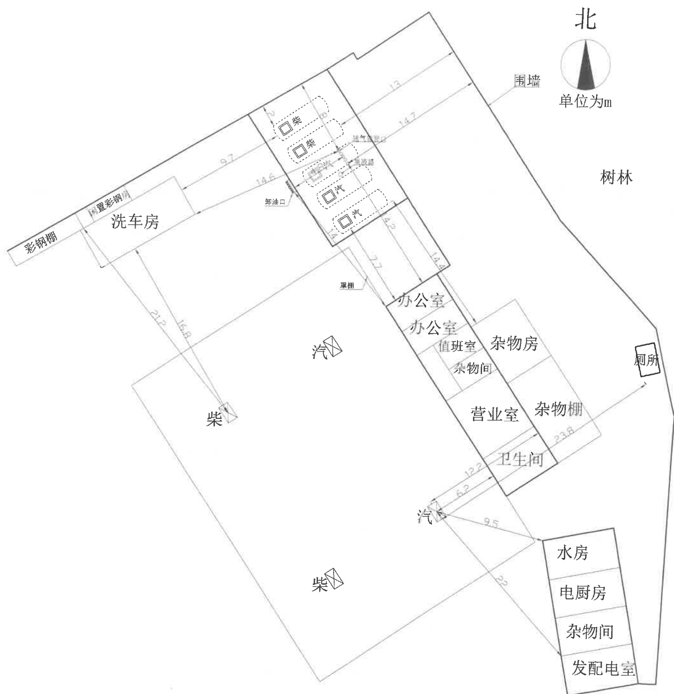
曲阳县定龙加油站平面布置示意图
